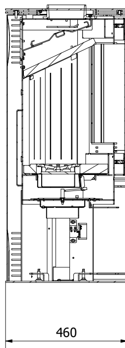
A-A ( 1 : 10 )
