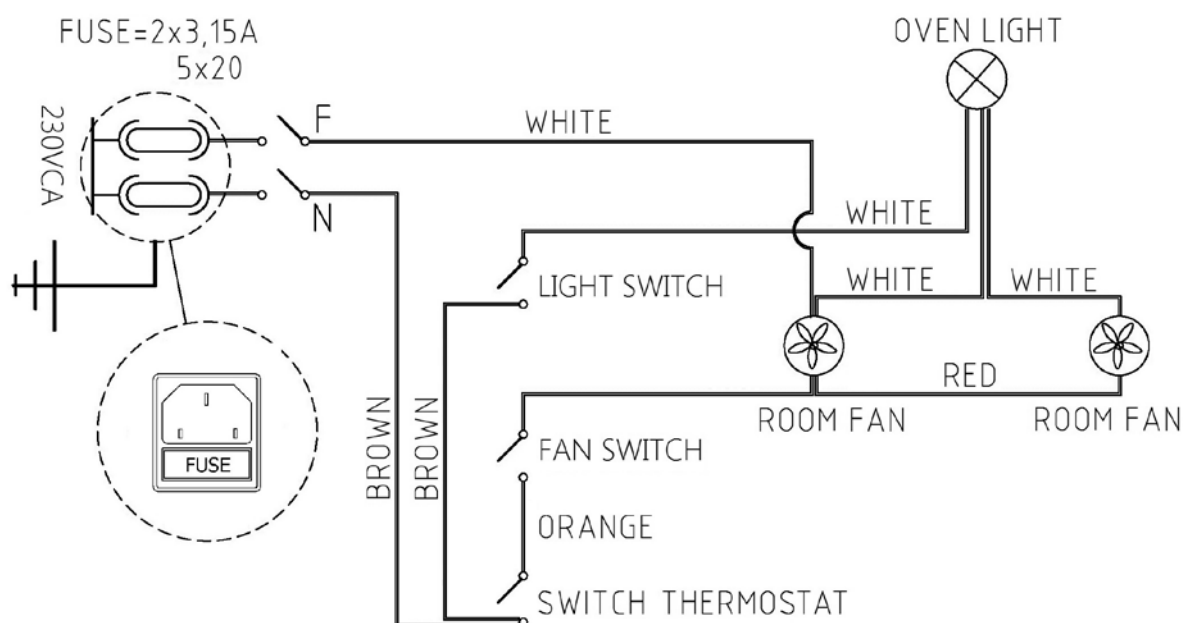
Fig. 83 - Schema électrique
