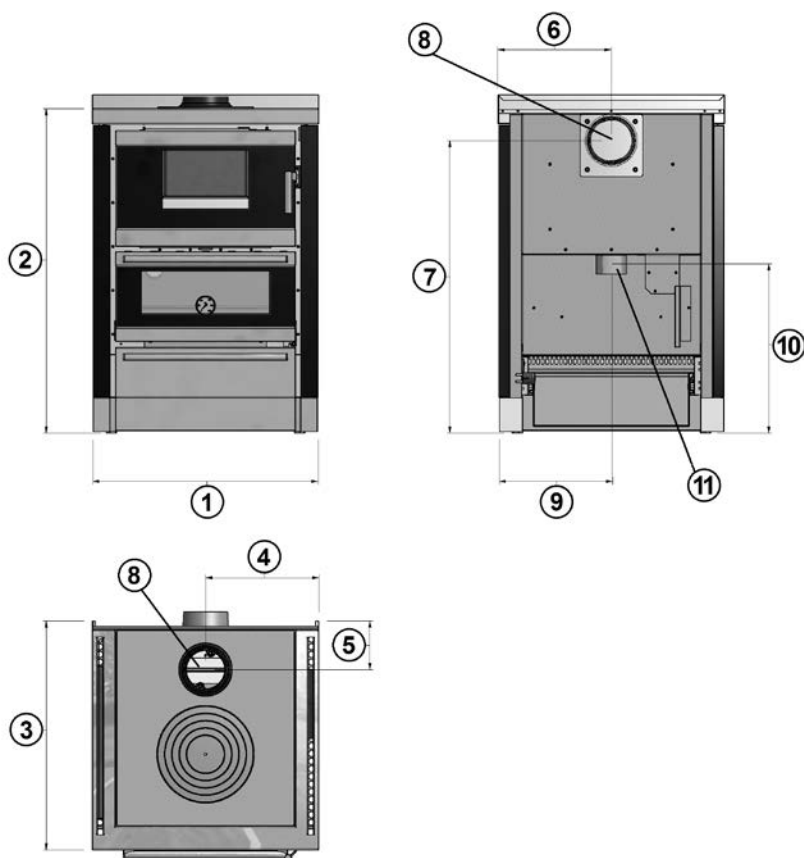
Fig. 10 - Dimensions générales: Kook 60 4.0 - Kook 67 4.0 - Kook 70 4.0
