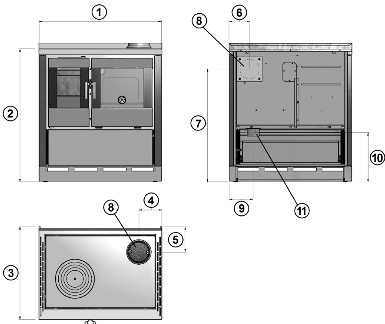
Fig. 11 - Dimensions générales: Kook 80 - Kook 87 - Kook 90 4.0
