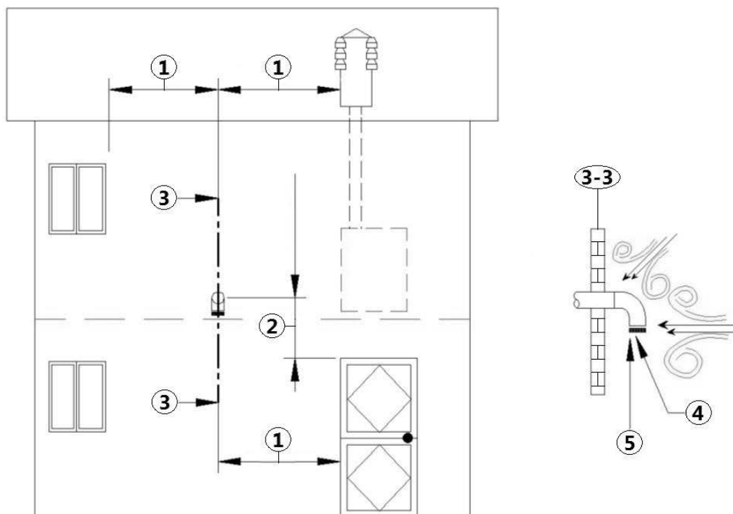
Fig. 6 - Air comburant
