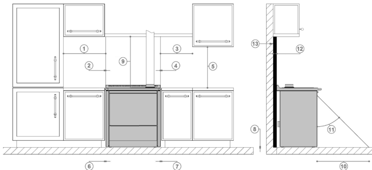
Fig. 15 - Installation à encastrement
